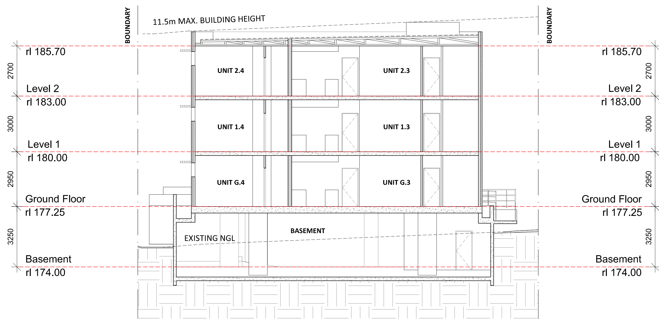
section A-A
