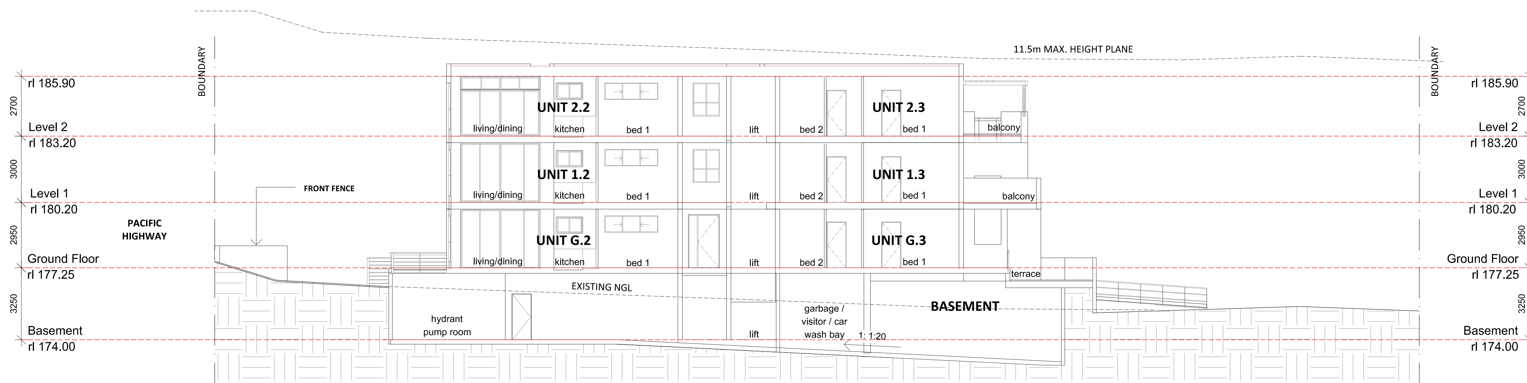
section D-D
